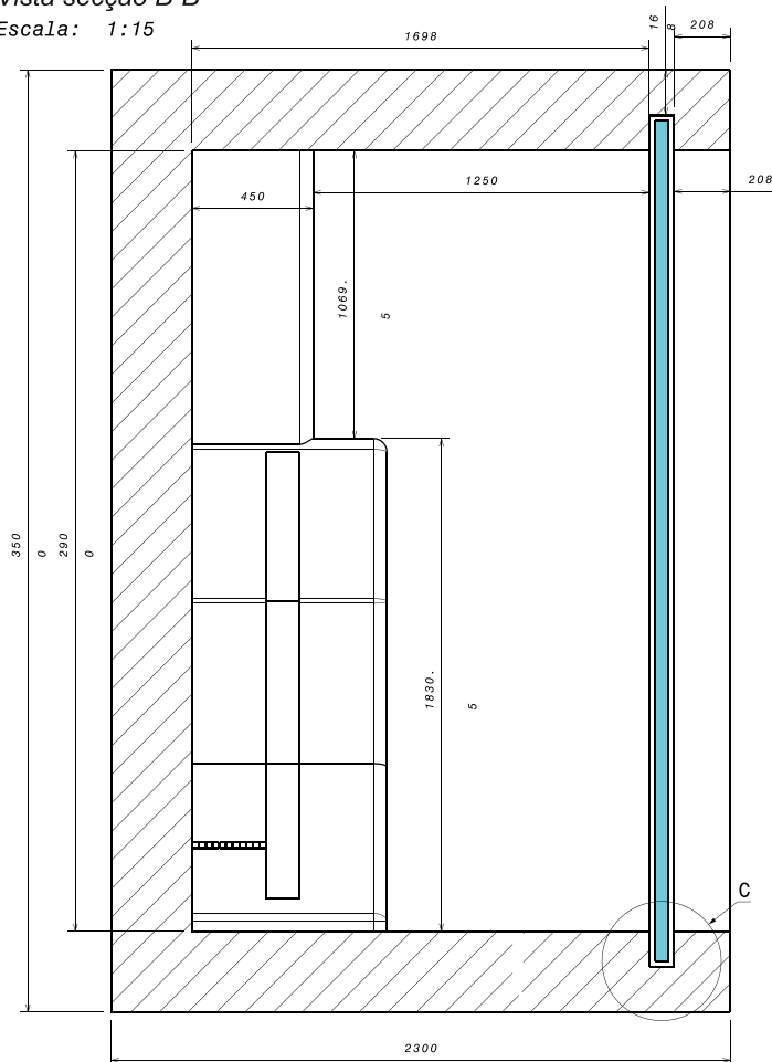
Vista secção B-B
