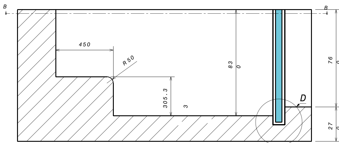
Vista secção transversal
