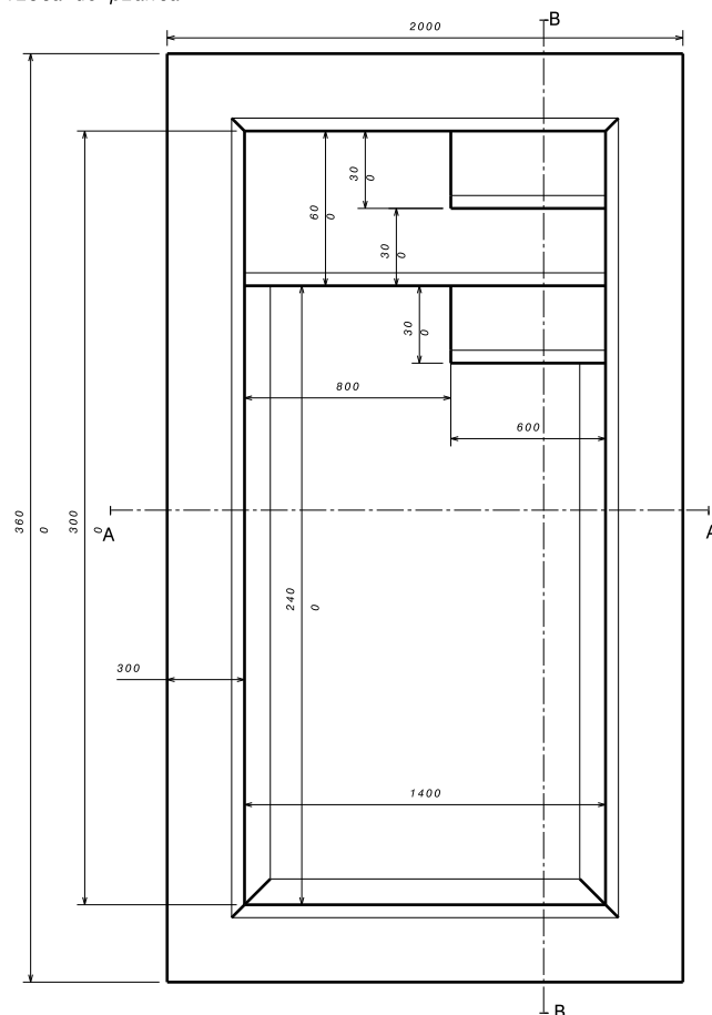
Vista de planta
